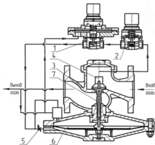
Регулятор давления РДБК-1
