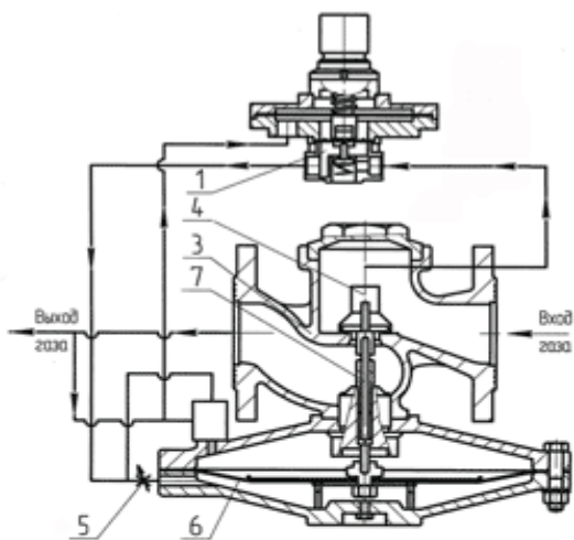
Регулятор давления РДБК-1П
